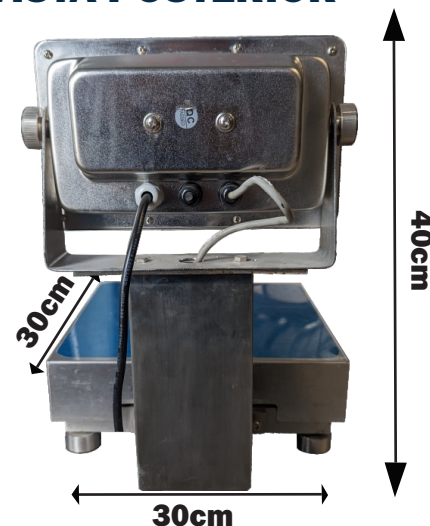
VISTA POSTERIOR
